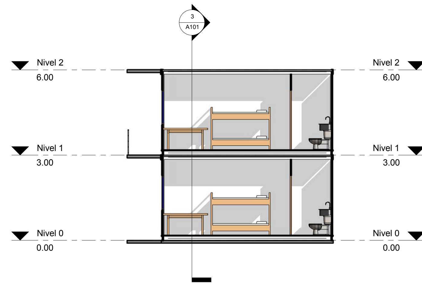
1 Sección Transversal 1 1 : 75
