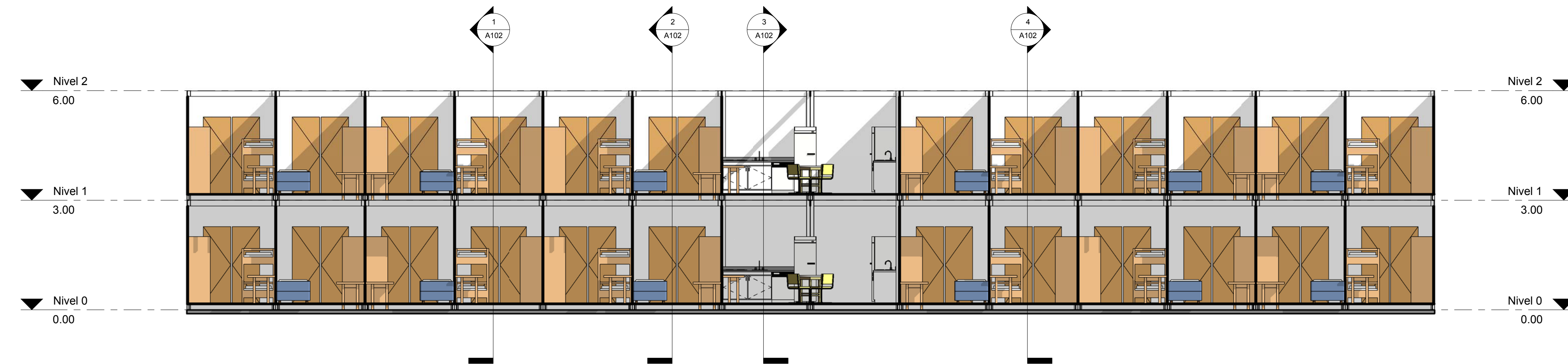
3 Sección Longitudinal 1 : 75
