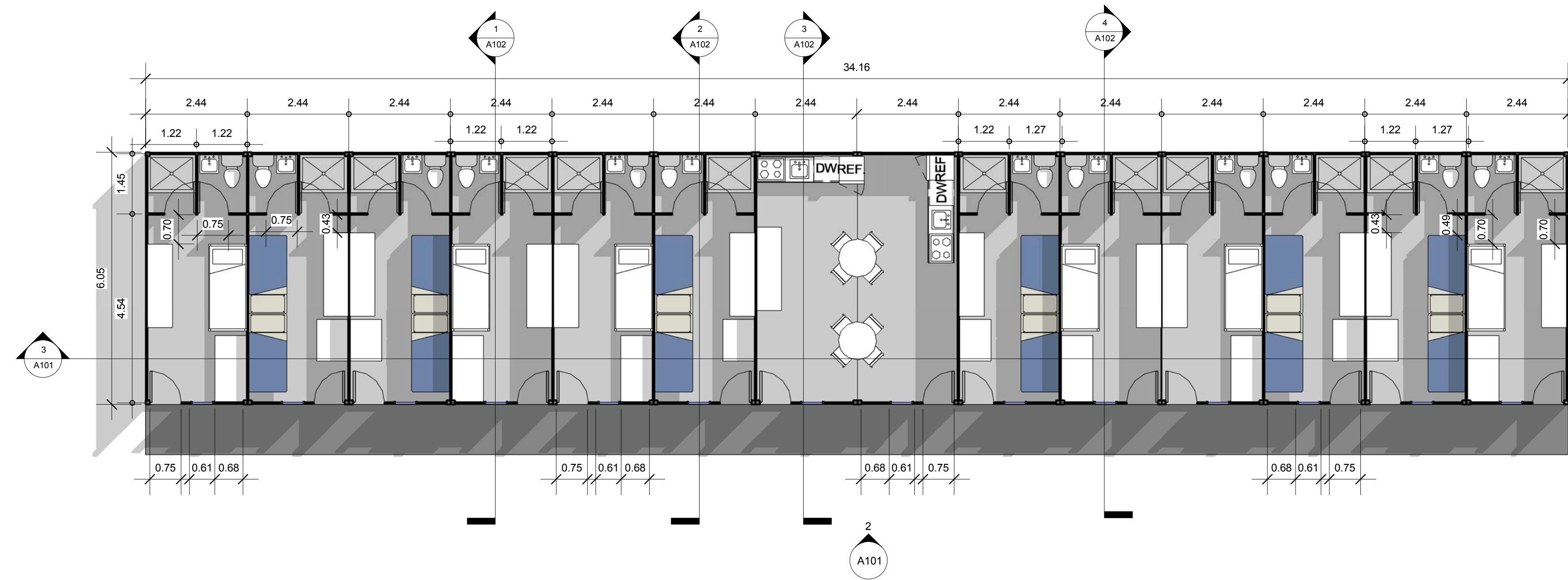
1 Planta Tipo 1 : 75
