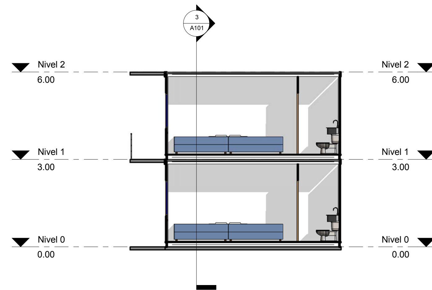
2 Sección Transversal 2 1 : 75
