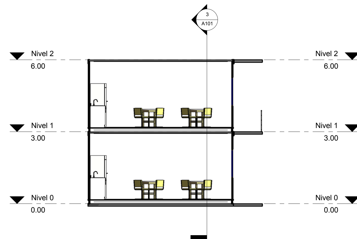
3 Sección Transversal 3 1 : 75
